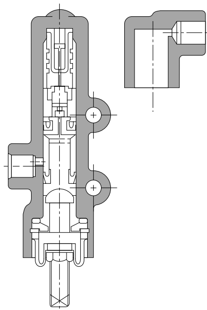
CILINDRO MESTRE SECUNDÁRIO
