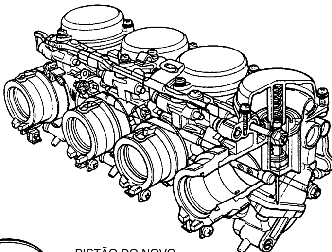
PISTÃO DO NOVO CARBURADOR TIPO VP
