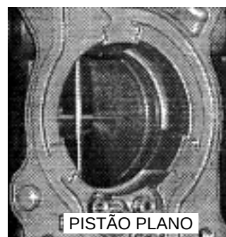
PISTÃO DO NOVO CARBURADOR TIPO VP
