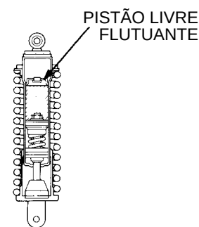
AMORTECEDOR TIPO DECARBON
