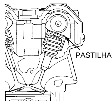
TIPO EMPUXO DIRETO
