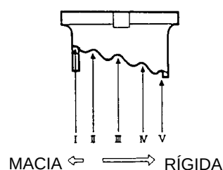
AJUSTADOR TIPO CAME
