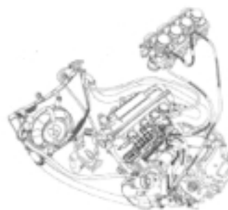
FLUXO DO LÍQUIDO DE ARREFECIMENTO (FRIO)
