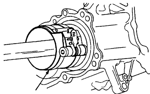
CINTA COMPRESSORA DE ANÉIS (FERRAMENTA CONVENCIONAL)
